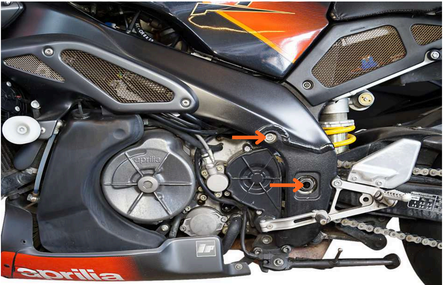
Montaż na pojeździe / Montering vid fordonet
