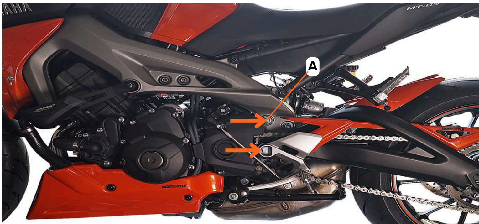
Montaż na pojeździe / Montering vid fordonet
